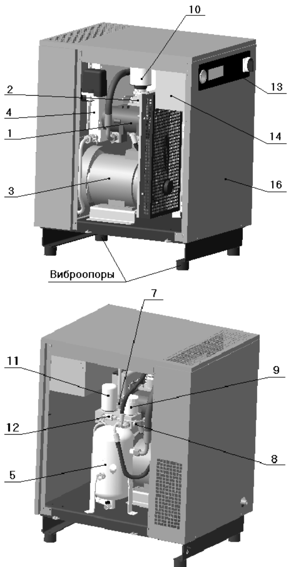
Рисунок 1 – Общий вид компрессорной установки VK5E-..., VK7E-..., VK10E-...
