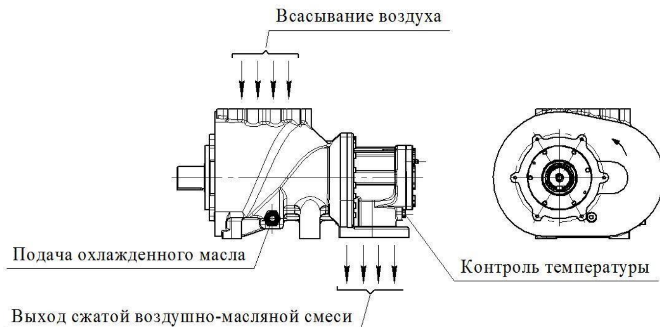
Общий вид блока винтового ITA23DR:
